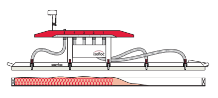
Einblasplatte Für das Dämmen oben offener vorgefertigter Holzbau-elemente (im Werk).
